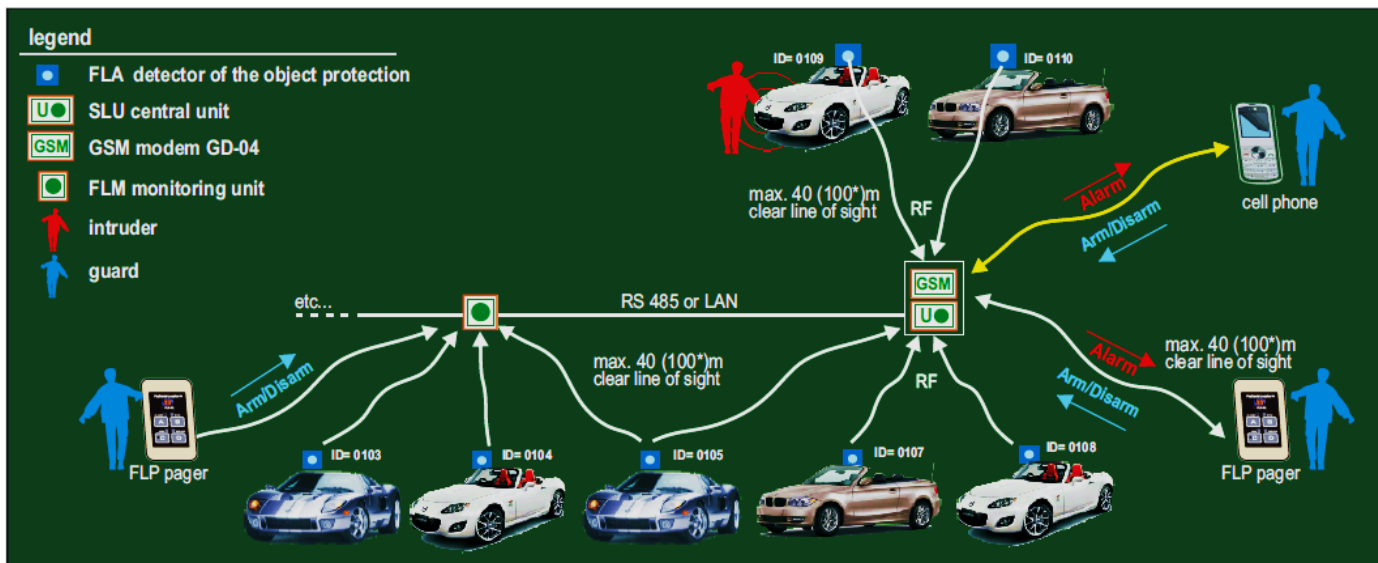
Systemarchitektur mit GSM- Modem und mehreren FLM Einheiten Radius > 50m
