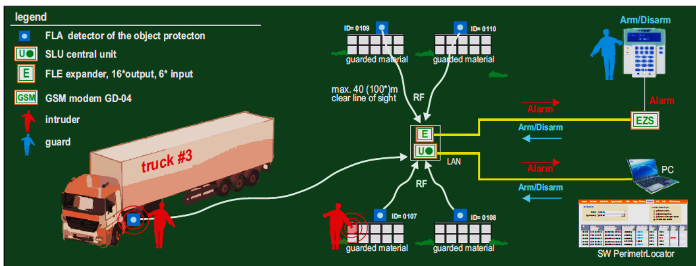
Fig. 1 – Systemarchitektur mit einer Alarmanlagenzentrale
