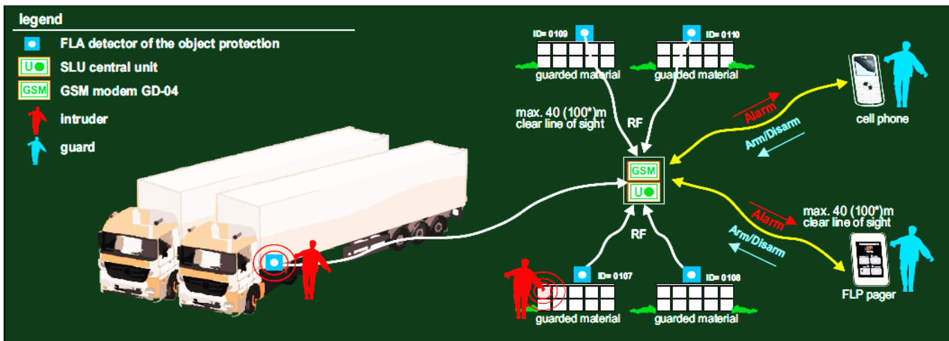
Systemarchitektur mit GSM- Modem – Radius bis zu 50m
