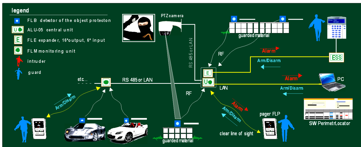
Systemarchitektur mit Computer oder Alarmanlage und mehreren FLM Einheiten
